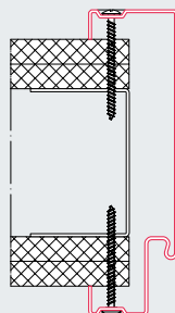
Obvodová stavební zárubeň pro hrázděné zdivo Profil 21120 s upevněním zrcadlovými šrouby
