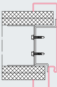
Obvodová zárubeň pro hrázděné zdivo Profil 21120
