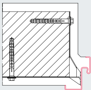
Rohová zárubeň DIN 18111 pro zdivo Profil 11100 i jako obvodová zárubeň, profil 21100
